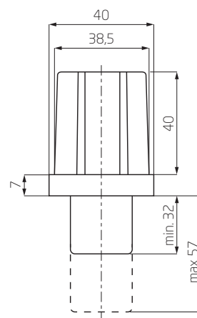
Stopka ze stali nierdzewnej do profilu 40x40 mm
