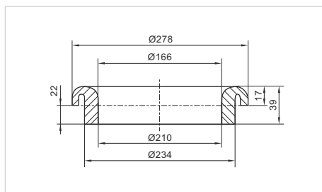
KP-DG-6 GREEN
