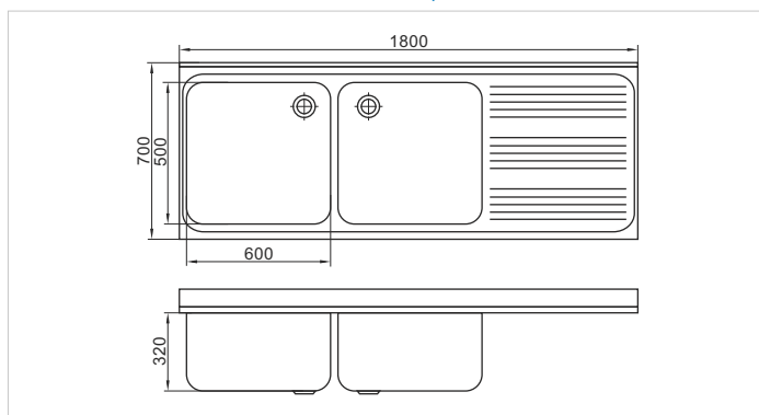
KZ-180706532/2L
