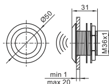
AG-3015N
