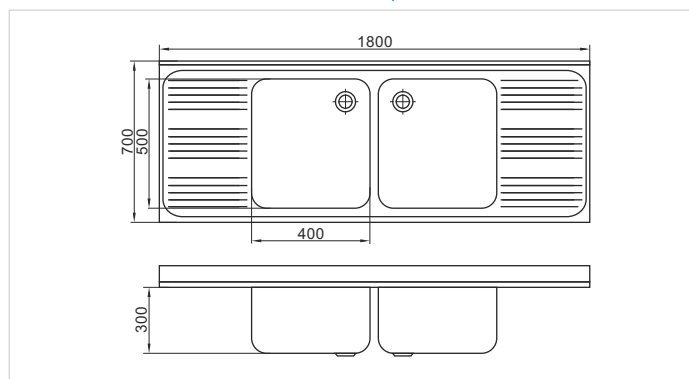
KZ-180705430/2LP
