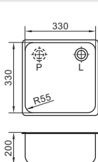
KZ-333320M
