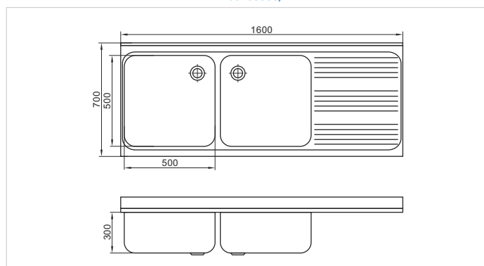
KZ-160705530/2L
