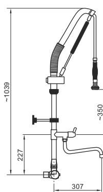
AG-PCP
