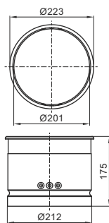
KP-CP-20-24AR
