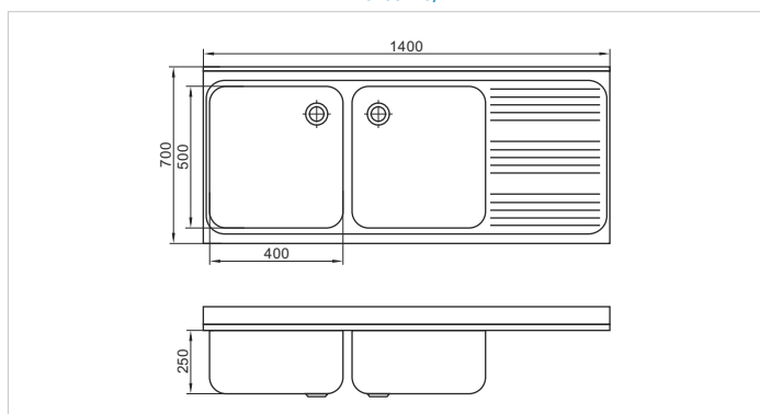
KZ-140705425/2L
