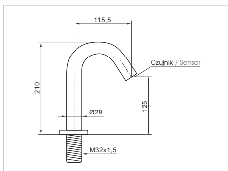
AG-3015N
