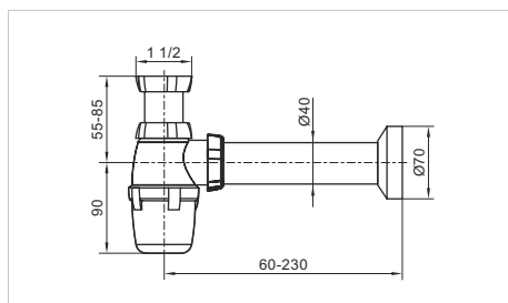
SYFON 1 1/2" BOTTLE TRAP 1 1/2"
