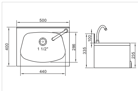
WYMIARY DIMENSIONS
