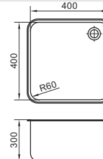
KZ-404030M
